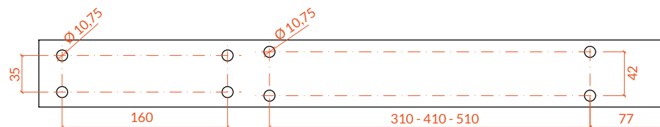
RZUT ODGÓRNY
