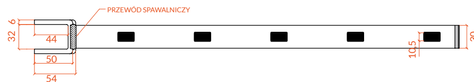
RZUT ODGÓRNY
