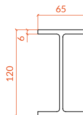
PROFIL
