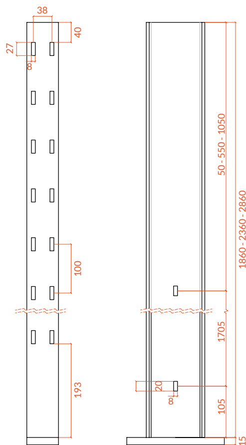
PROFIL
