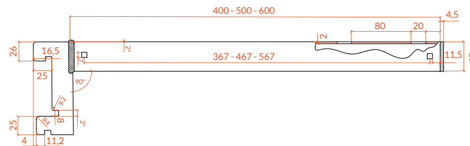
RZUT PRZEDNI
