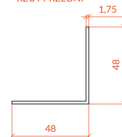
RZUT ODGÓRNY
