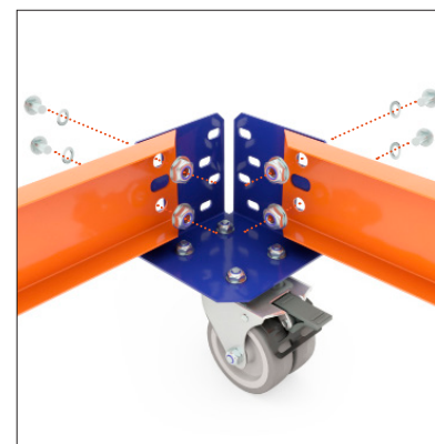
Sposób łączenia trawersów do płytki Śruby 10 mm
