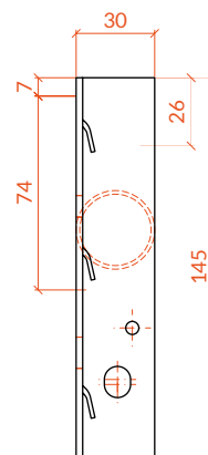
PROFIL
