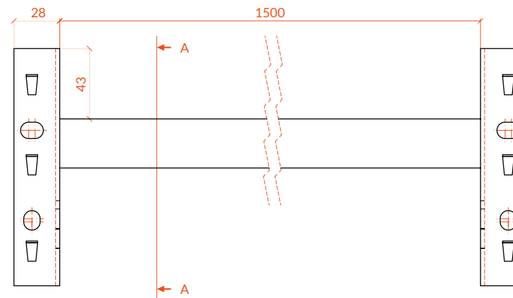
RZUT PRZEDNI
