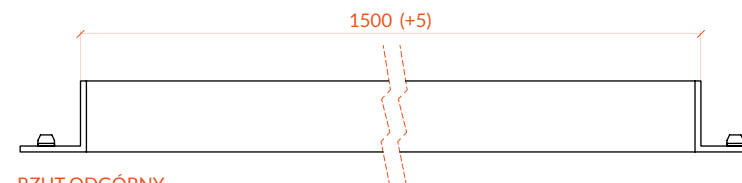
RZUT ODGÓRNY
