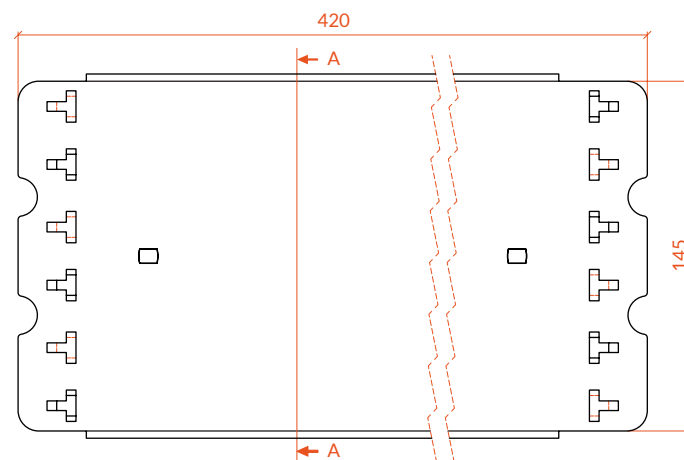
RZUT PRZEDNI
