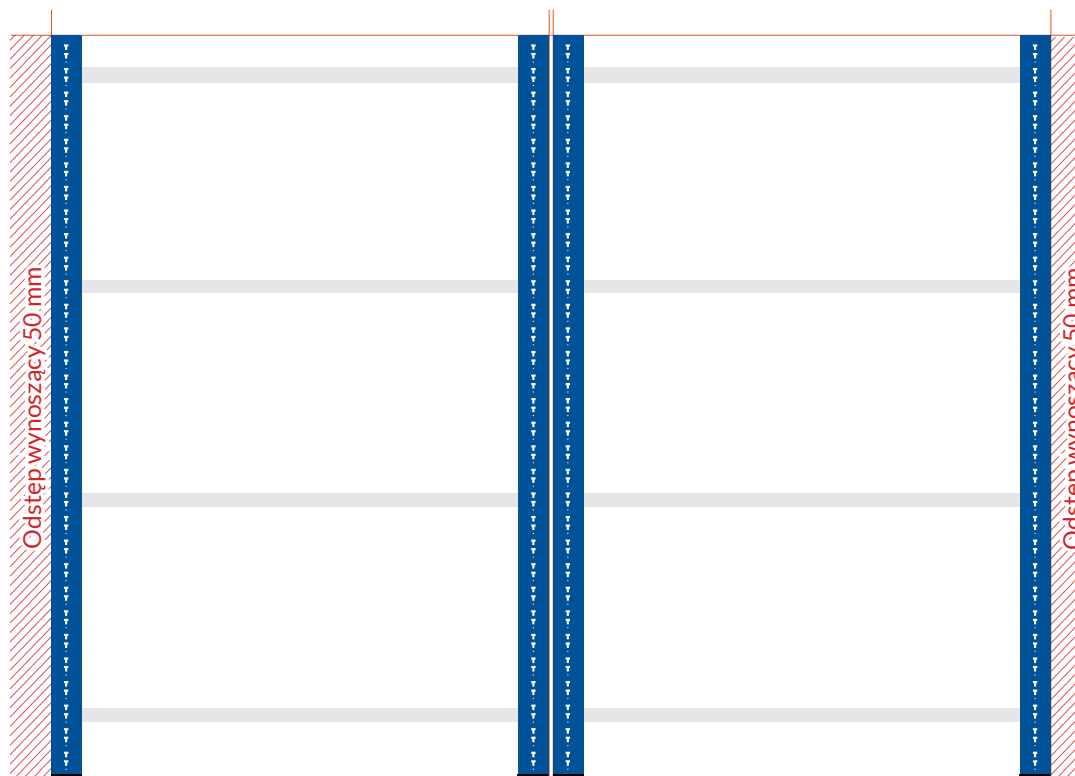
CIĄG REGAŁÓW
