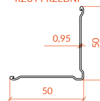
RZUT ODGÓRNY
