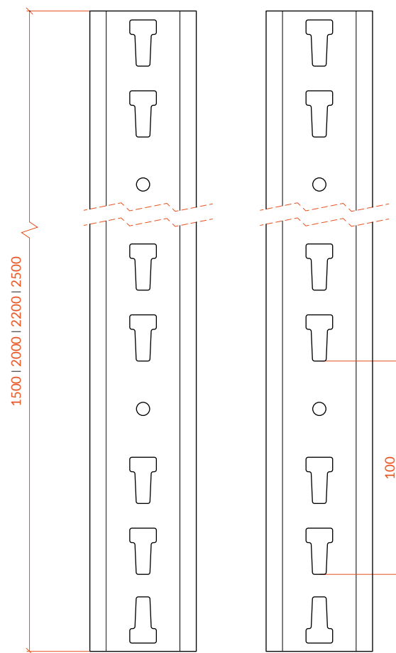
PROFIL
